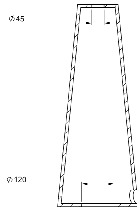
SECTION AG-AG
